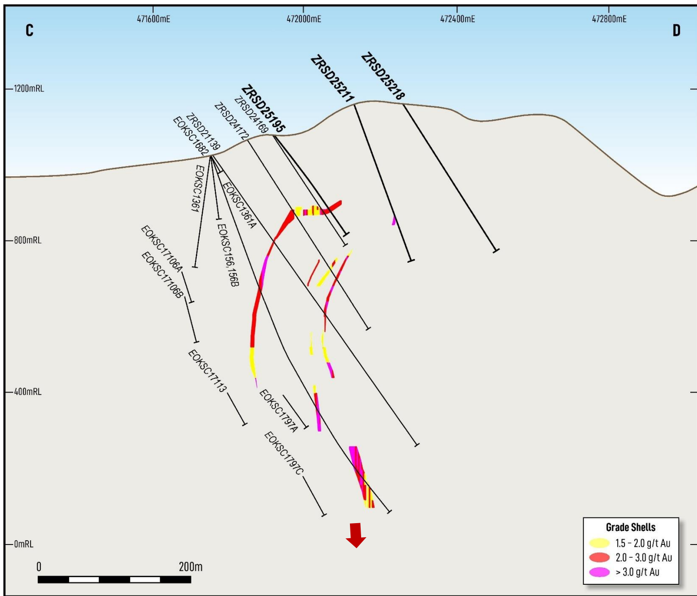
Slika 5. Gradina – poprečni presek C–D, pogled ka severu, sa trasama bušotina i blokovima modela >1,5 g/t Au.
