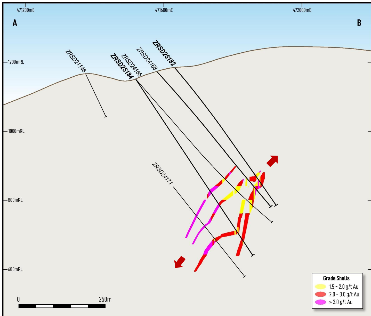
Slika 4. Poprečni presek Gradine duž A – B, gledajući ka severu, sa tragovima bušenja i modelnim blokovima >1.5 g/t Au.
