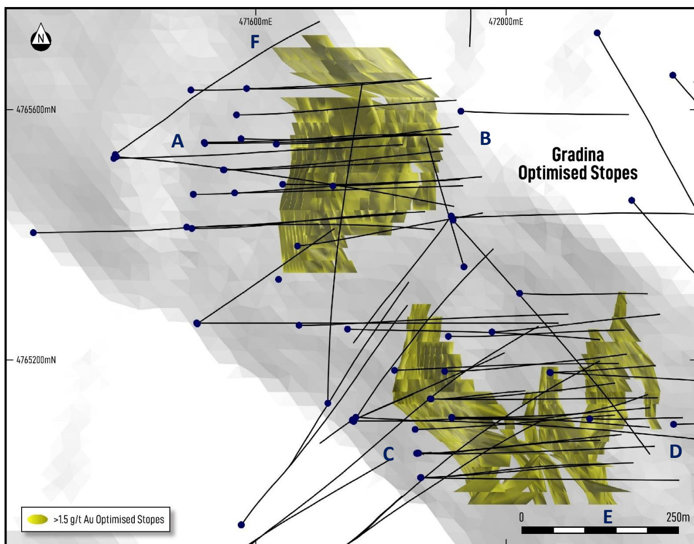
Slika 3. Mapa Gradine koja prikazuje tragove bušenja i otisak ležišta (>1,5 g/t Au optimizovane stope), sa pozadinskom topografijom i oznakama profila za naredne slike.
