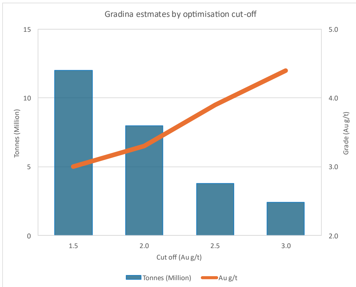
Slika 2. Odnos sadržaja i tonaže pri otvorenom podzemnom otkopavanju sa dubinskim bušenjem na nalazištu Gradina.
