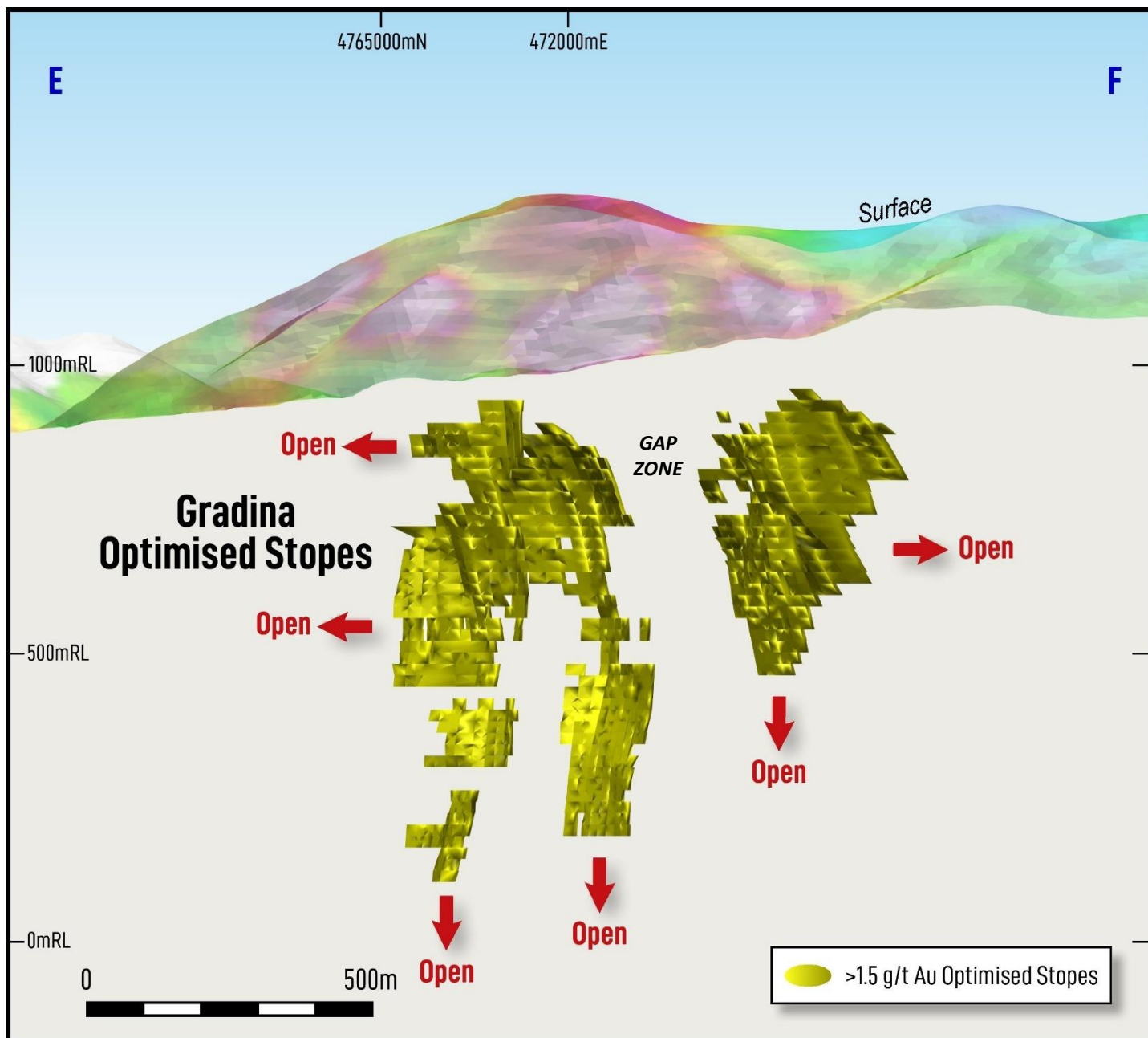
Slika 6. Poprečni presek Gradine duž E – F, gledajući ka jugozapadu, prikazuje optimizovane podzemne otkope sa geohemijskom anomalijom zemljišta zlata i arsena prikazanim preko topografije.
